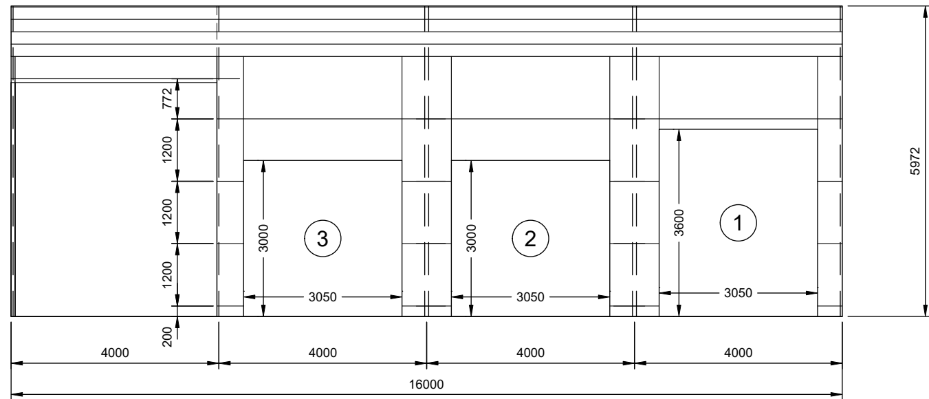
2 LEFT ELEVATION 3 SCALE: 1:100
