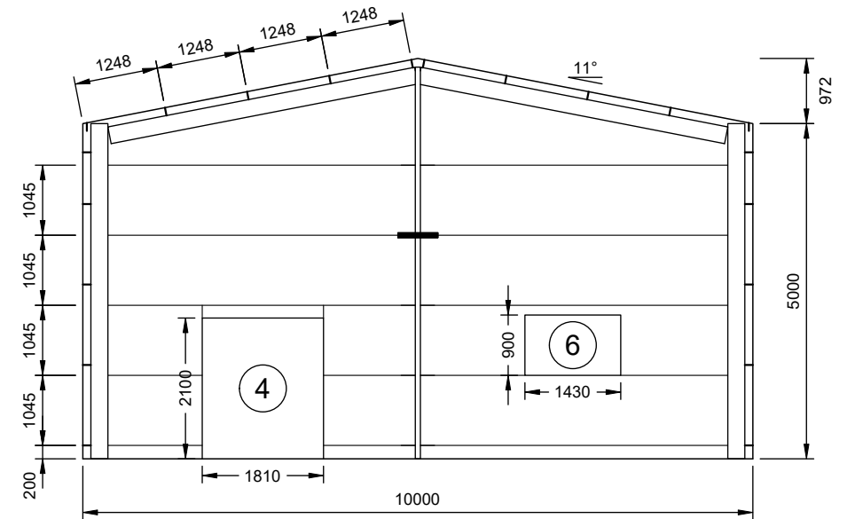
3 REAR ELEVATION 3 SCALE: 1:100 FRAME #4
