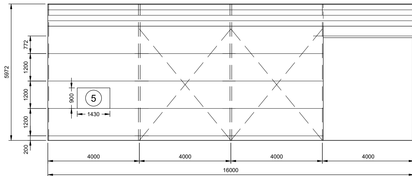
1 RIGHT ELEVATION 3 SCALE: 1:100
